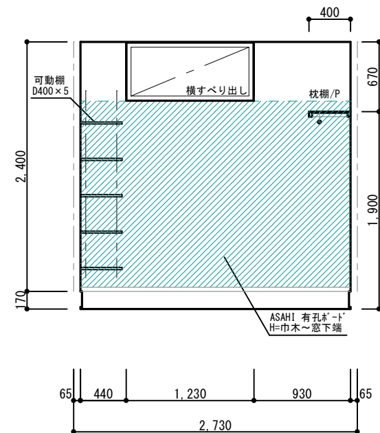
SC 東面
