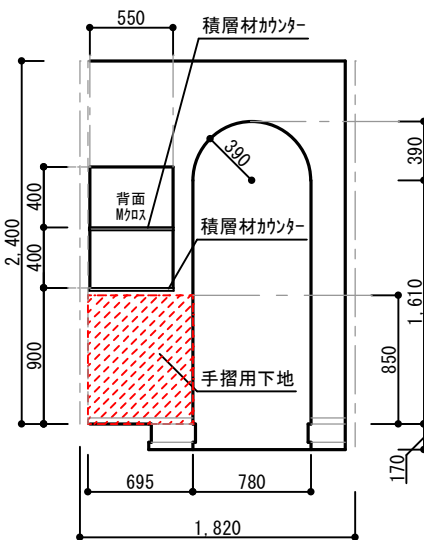
玄関 東面
