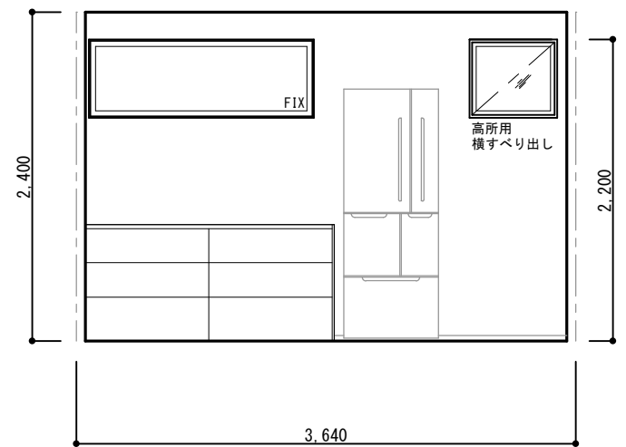
LDK 北面
