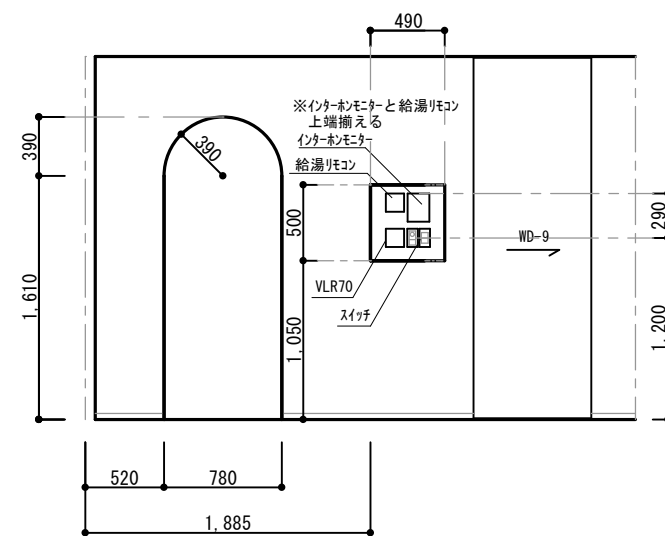
LDK 東面
