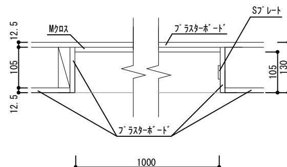
キッチン ニッチ 上部断面図
