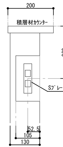
キッチン ニッチ 断面図
