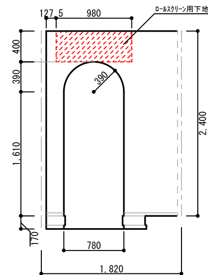
SC 東面
